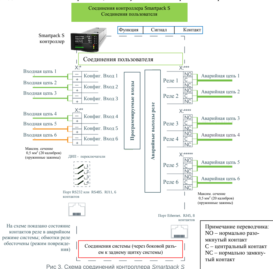
Рис 3. Схема соединений контроллера Smartpack S
