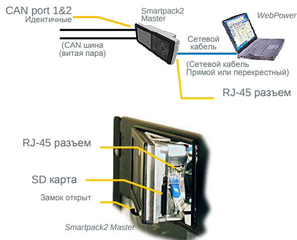
Рис 2 Расположение портов CAN ports и Ethernet разъема в контроллере Smartpack2 Master
