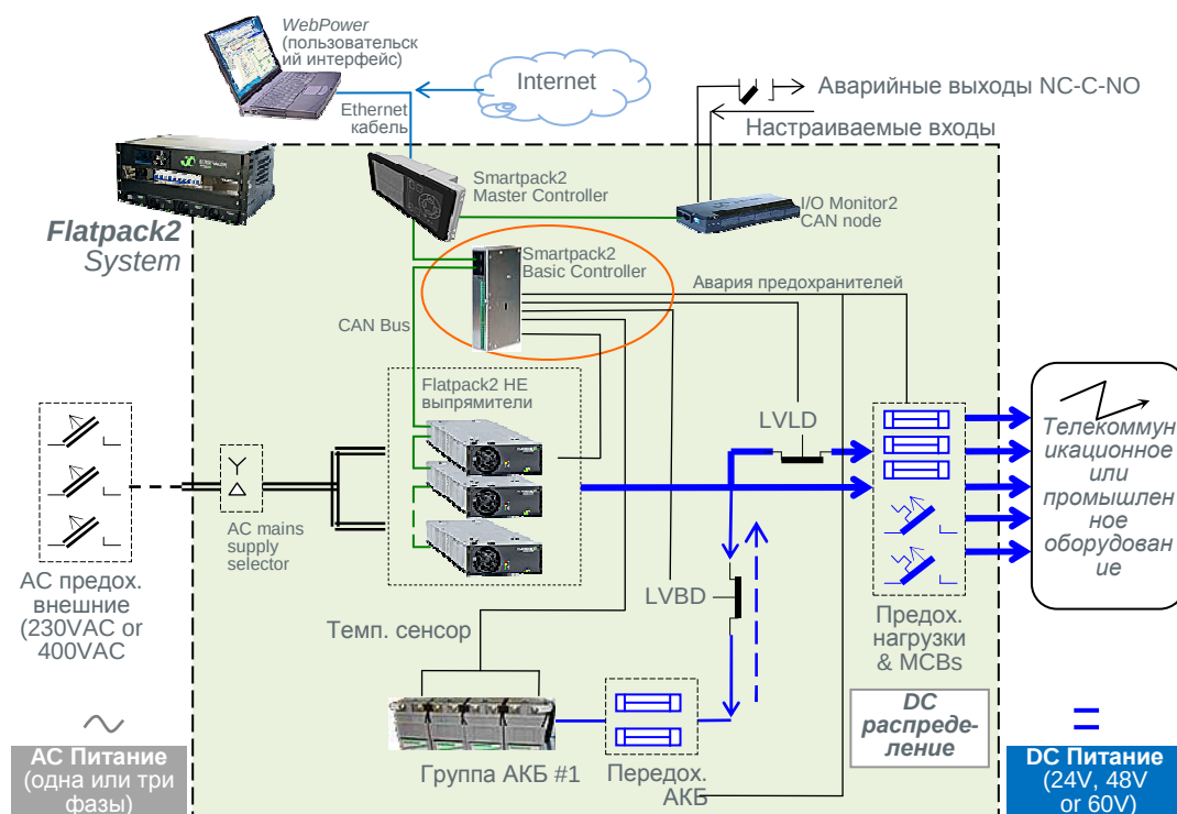
Рис1 стандартная система постоянного тока Flatpack2 для телекоммуникационной и промышленной отраслей, питающаяся от внешних источников электропитания. Состоит из выпрямителей, расположенных на полках, одного мастер контроллера и одного основного контроллера, системы распределения постоянного тока и т.д.
